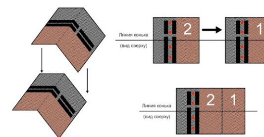
Рис. 32. Устройство ребер скатов и коньков.
