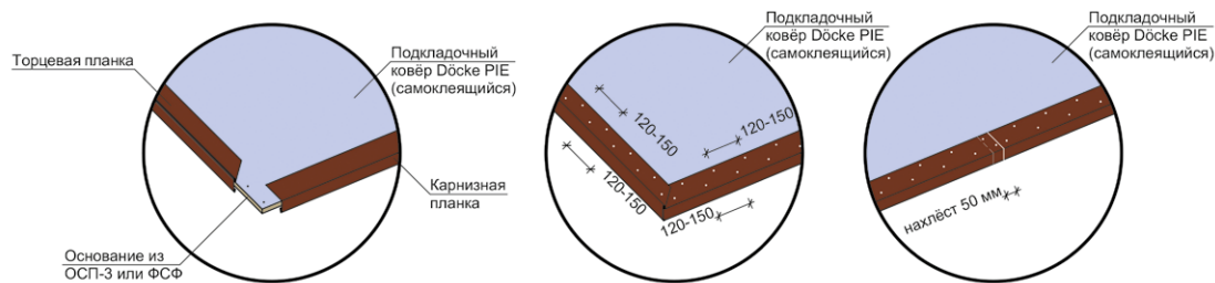
Рис. 13. Крепление металлических карнизных и торцевых планок.
